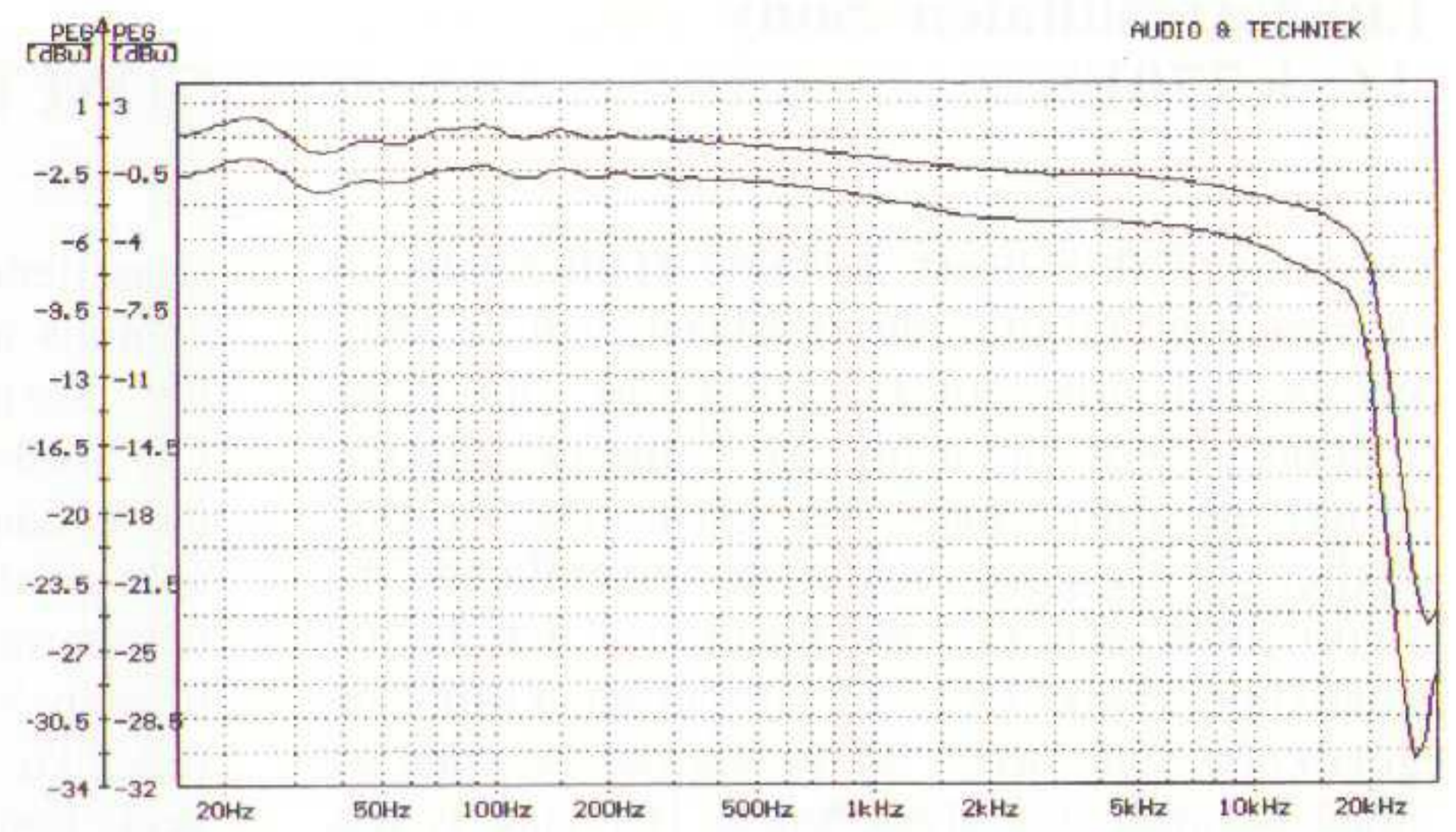
Akai GX-67
